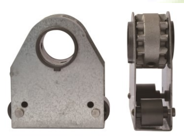
L001开窗齿轮 材质：镀锌钢板 适用齿条高度：30mm L001 Ventilation gear Material: Galvanized steel Applicable height: 30mm
